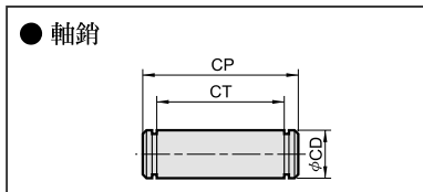
外形尺寸表
