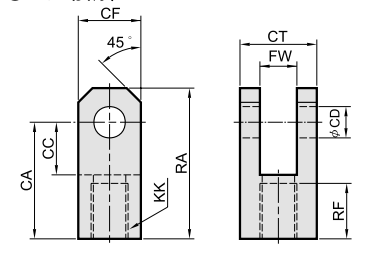
外形尺寸表
