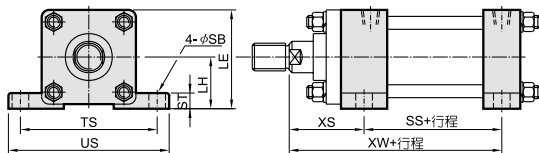
外形尺寸表
